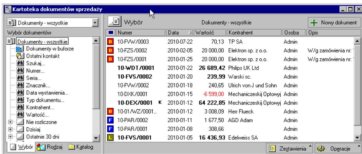
Rys. 2-2 Okno kartoteki dokumentów sprzedaży.
