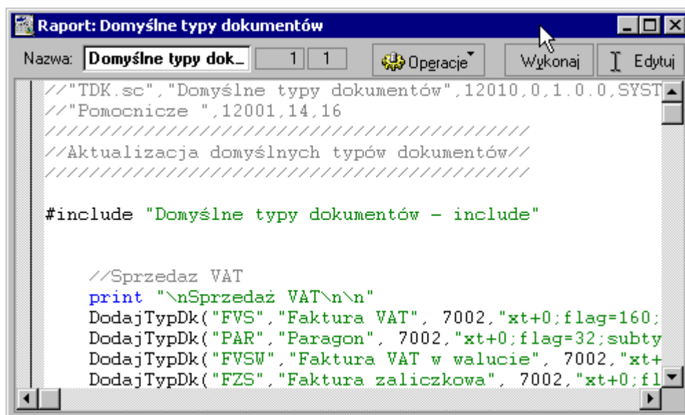
Rys. 2-4 Okno edytora raportów.
