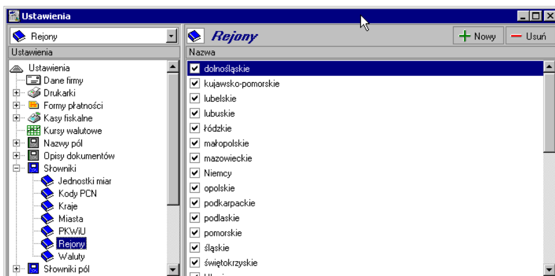
Rys. 4-17 Przykład okna słowników.
